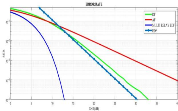
Fig.2: SER VS SNR
