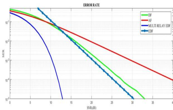
Fig.2: SER VS SNR
