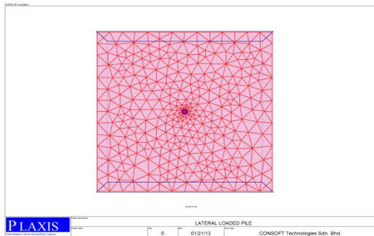
Fig: 5.1 2D Mesh
