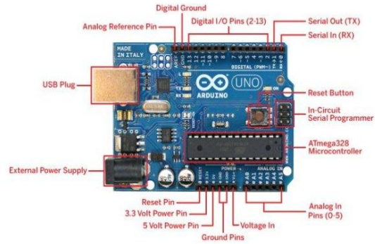
Fig.1. Arduino Uno
