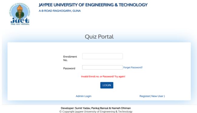
Fig. 4 Login Page
