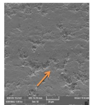
Fig 4d : 0.4wt% Al-G
