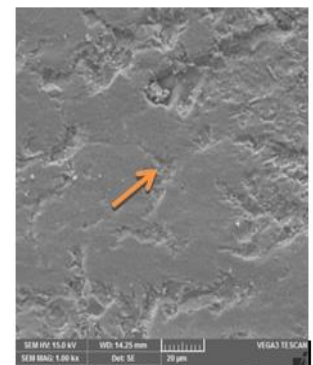
Fig 4b : 0.2wt% Al-G
