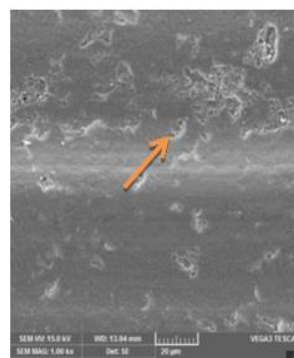
Fig 4c : 0.3wt% Al-G
