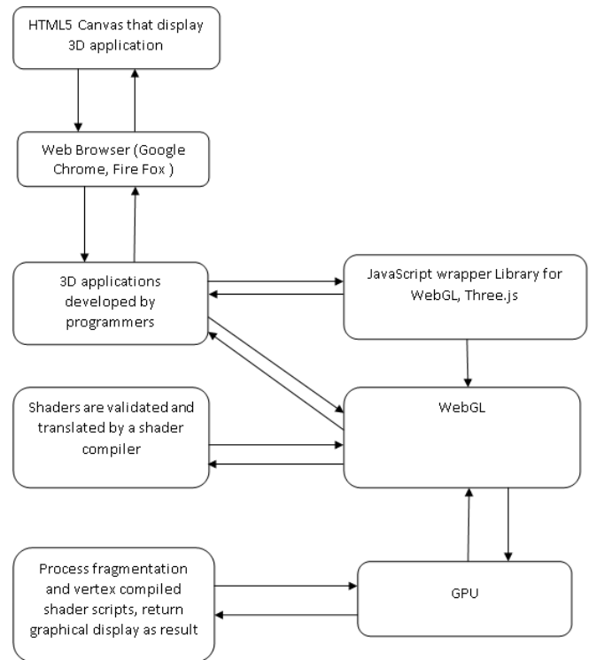
Fig 1.WebGL Stack[4]
